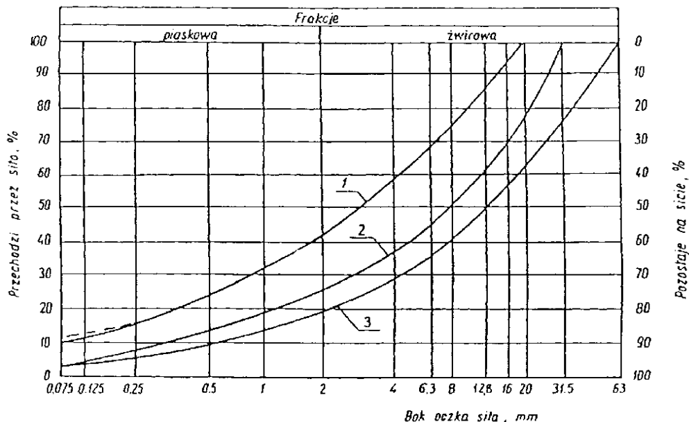
Rys. 1. Pole dobrego uziarnienia kruszyw dla podbudowy
