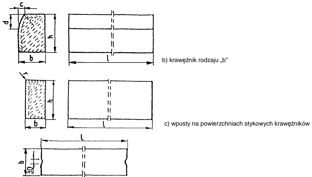
Rys. 1. Wymiarowanie krawężników Tablica 1. Wymiary krawężników betonowych
