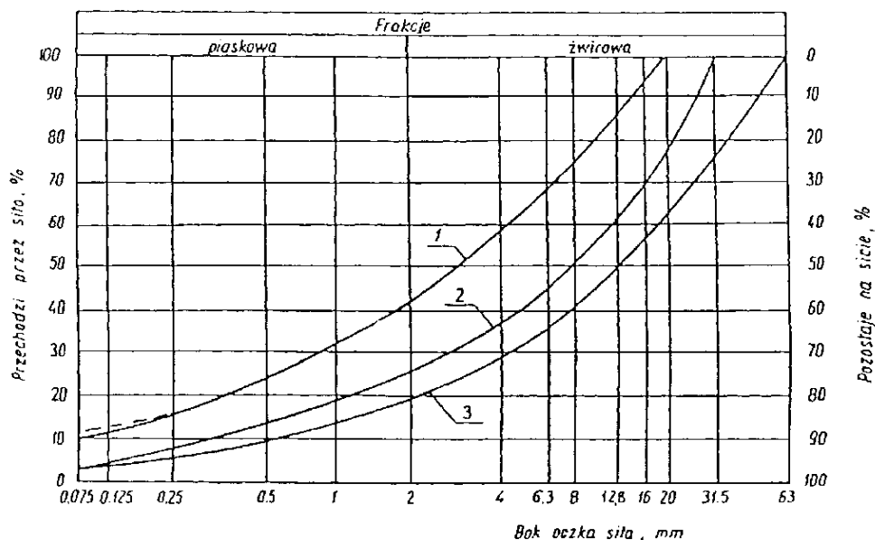
Rys. 1. Pole dobrego uziarnienia kruszywa dla podbudowy
